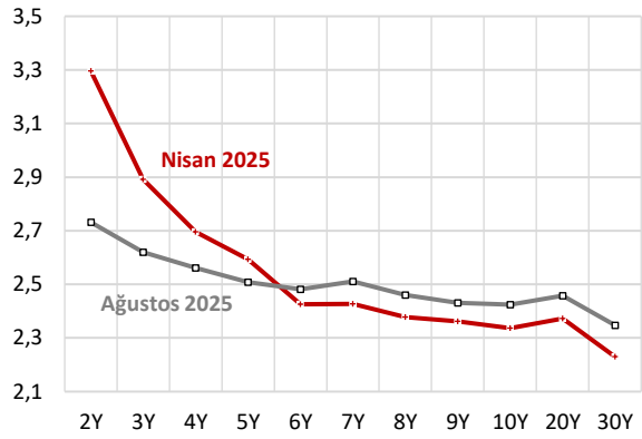
Grafik 12. ABD Başabaş Enflasyon Eğrisi (%)
