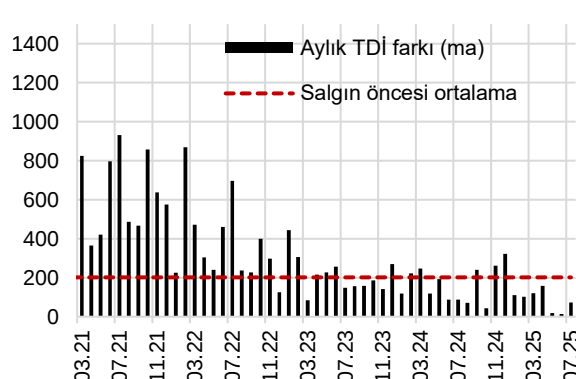
Grafik 10. Tarım Dışı İstihdam (TDİ, bin kişi)
