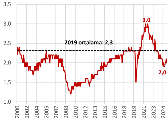
Grafik 14. İşten Ayrılma Oranı (Tarım Dışı, %)
