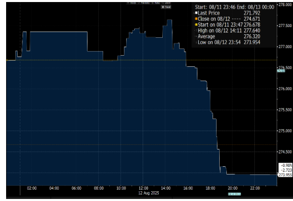
Grafik 8. Türkiye 5Y CDS Risk Primi
