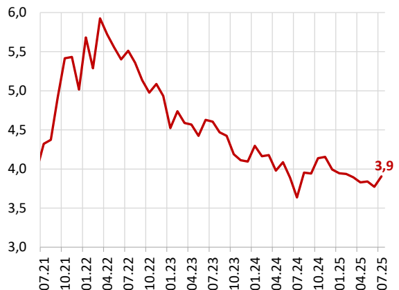
Grafik 16. Ortalama Saatlik Ücret (yıllık % değişim)
