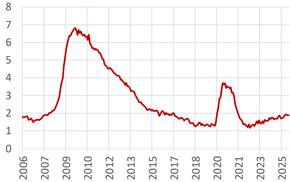
Grafik 20. İşini Kaybedenler (mevs. ard., milyon kişi)
